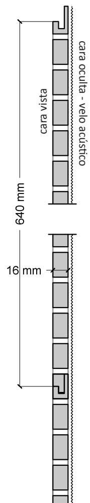
Sección transversal
